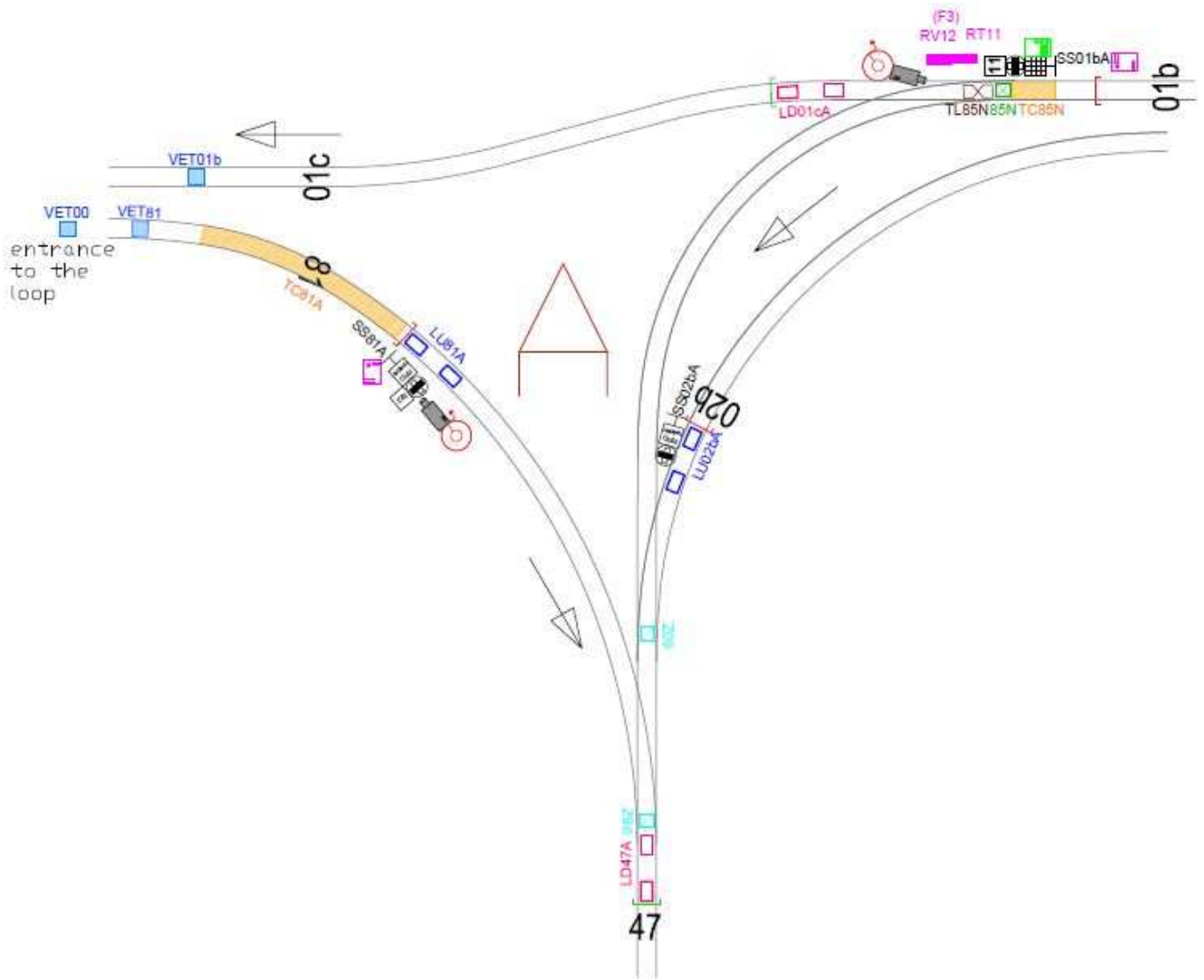
Zał. nr 1.3: Odcinki torowe w strefie A
