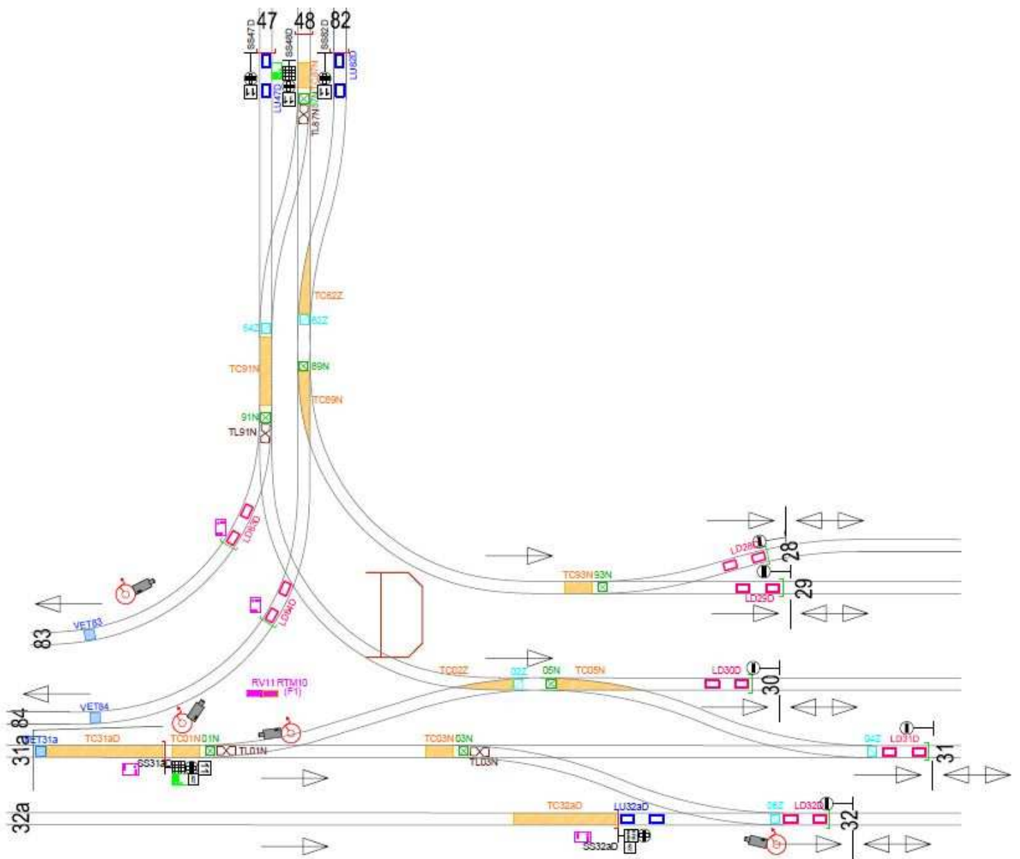
Zał. nr 1.5: Odcinki torowe w strefie D
