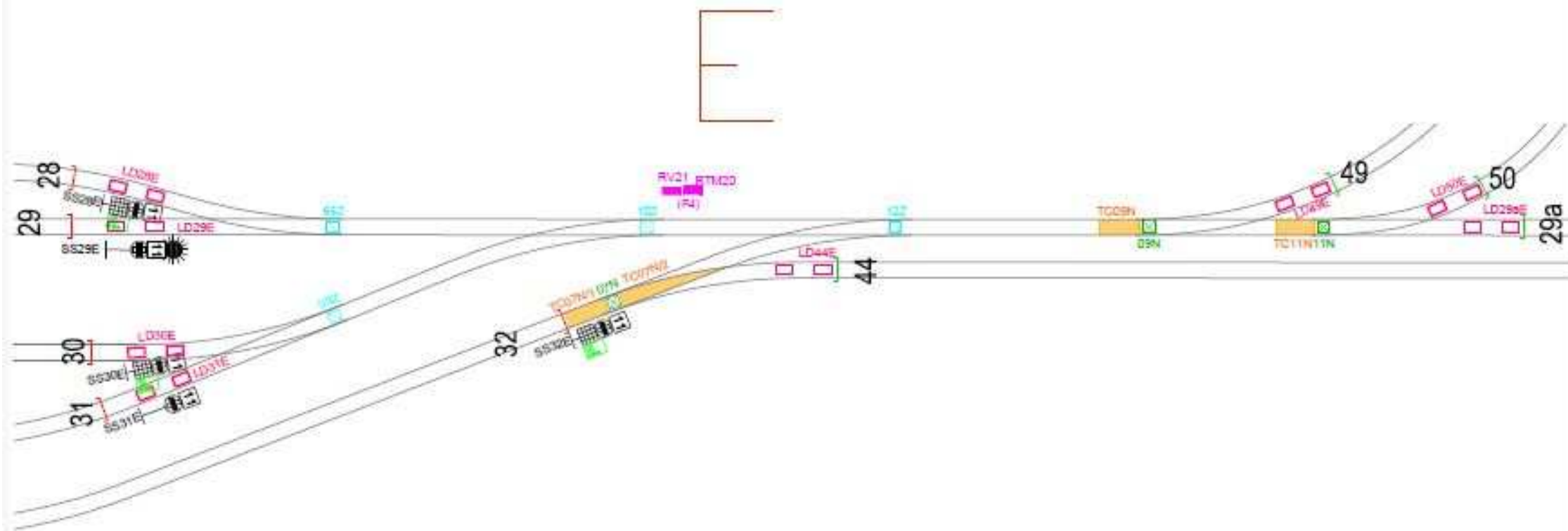
Zał. nr 1.7: Odcinki torowe w strefie E
